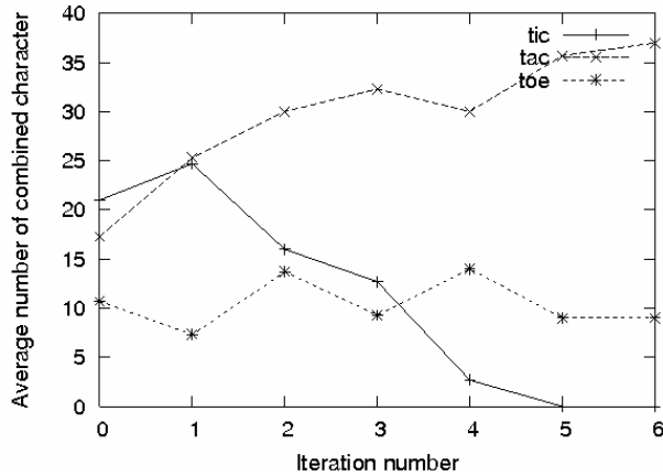
그림 2. 'tac'이 표적 단어일 때.
