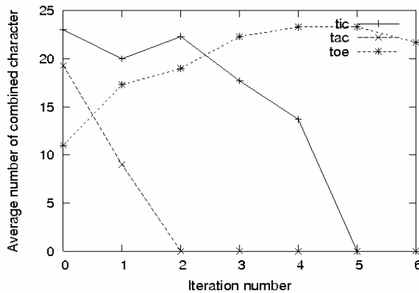
그림 3. 'toe' 가 표적 단어일때의 결과.
