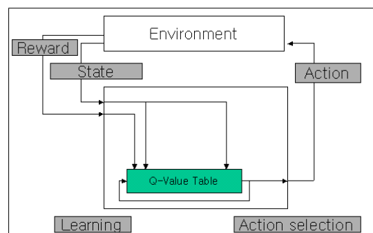
그림 1 . Q-Learning 모델
