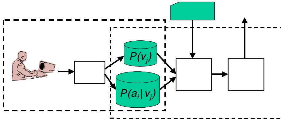
그림 1 감정 인식 엔진 TexMo의 전체 흐름도
