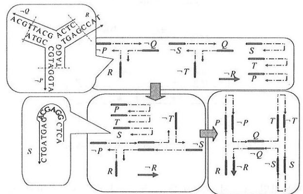
그림 1. 문제 "P ∧ Q → R, S ∧ T → Q, S, T, P, R?"에 대한 resolution refutation 과정의 모식도 (Preliminary Proc. of DNA8에서 발췌)
