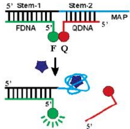
[그림 2] 구조 변화가 가능한 형광표지-앵타머 설계
