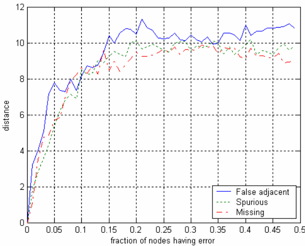
그림 2. 오류에 따른 허브 토폴로지의 거리 변화
